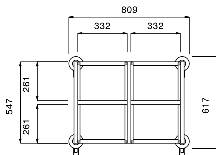
Boven aanzicht
